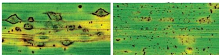
شکل ۶. برگ سمت راست حاوی سیلیس بیشتر و گسترش کمتر ضایعات بلاست (عکس از IRRI)
